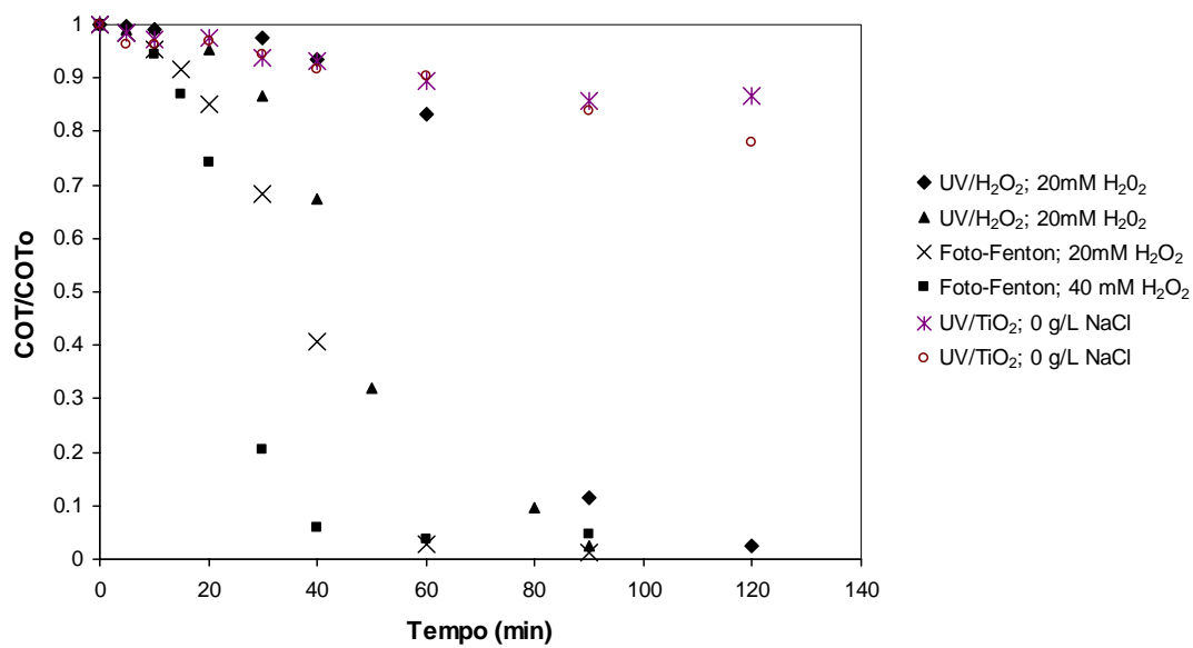
Figura 37 – Remoção de COT em função do tempo para algumas condições estudadas dos diferentes processos avaliados; [Fe(II)] = 0,2 mM; [TiO 2 ] = 1 g/L.
