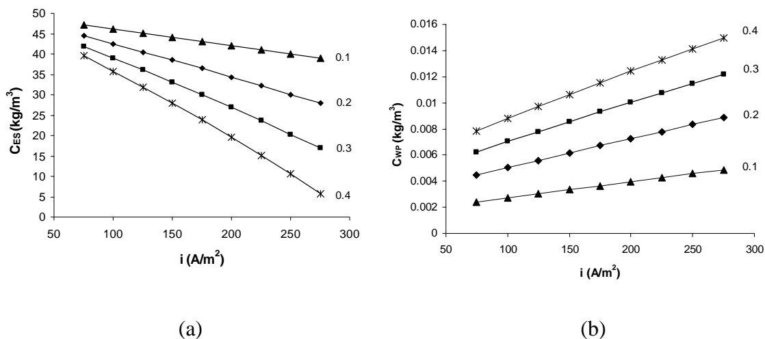
Figura 42 – Variação de C_{W_p} (a) e C_{E_s} (b) em função da densidade de corrente para diferentes valores de área de membrana ( m^2 ) em 30 minutos de operação.
