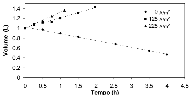
Figura 21 - Volume do compartimento do concentrado em função do tempo para diferentes valores de densidade de corrente aplicadas; [ \Delta C_s^0 \approx 55 \text{ kg} \cdot \text{m}^{-3} ; \Delta C_p^0 = 100 \text{ ppm C} ].
