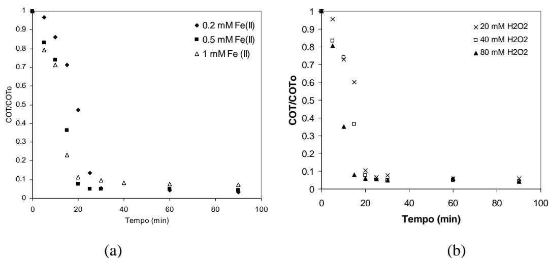
Figura 31 – Remoção de COT em função do tempo; (a) efeito da concentração de Fe(II), [H 2 O 2 ] = 40 mM; (b) Efeito da concentração de H 2 O 2 , [Fe(II)] = 0,5 mM.
