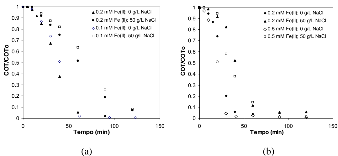
Figura 35 - Remoção de COT em função do tempo para as condições do planejamento experimental; efeito [Fe(II)] – processo foto-Fenton; (a) [\text{H}_2\text{O}_2] = 20 \text{ mM} ; [\text{H}_2\text{O}_2] = 40 \text{ mM} ; [\text{H}_2\text{O}_2] .
