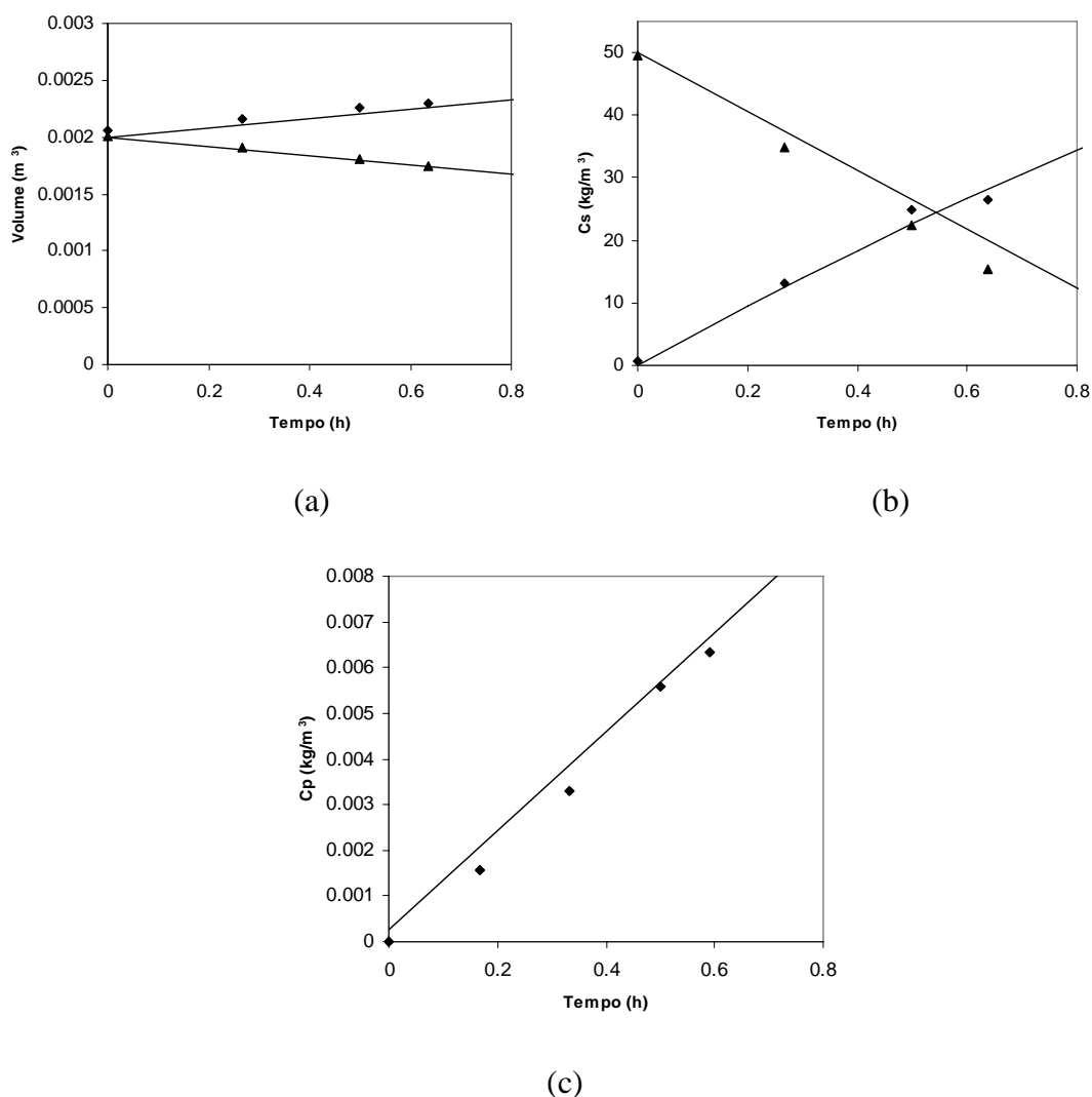
Figura 40 – Variação do volume (a), concentração de sal (b) e fenol (c) com o tempo nos tanques T_E e T_W ; predição modelo e valores experimentais; i=275 \text{ A/m}^2 .
