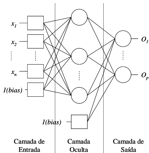
Figura 15 – Estrutura de uma rede neural artificial de tipo feedforward (Gob et al., 1999).
