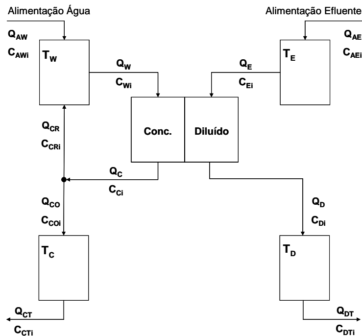
Figura 45 – Configuração do modelo contínuo com reciclo no concentrado ; Q : vazão das correntes; C : concentração; subscripto i : fenol e sal.
