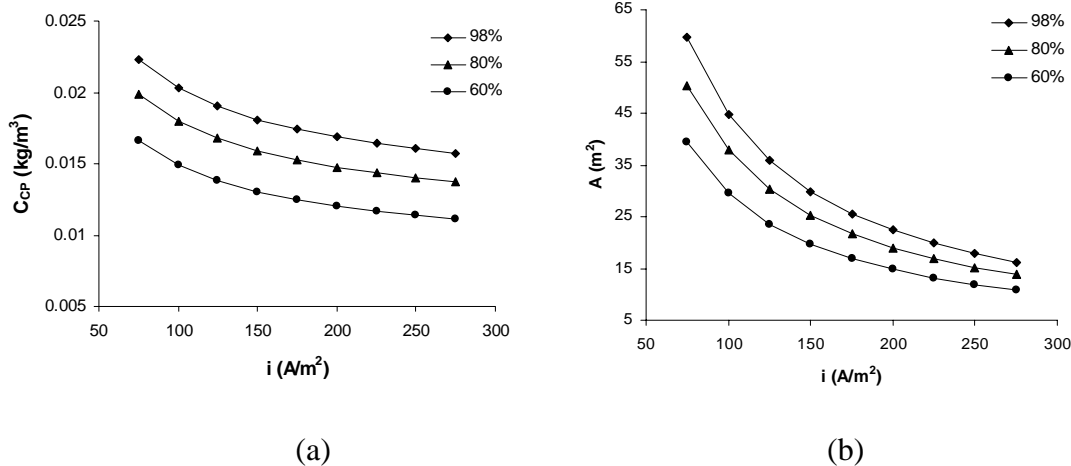
Figura 44 - Variação de (a) C_{C_p} e A (b) em função da densidade de corrente para diferentes percentuais de dessalinização.
