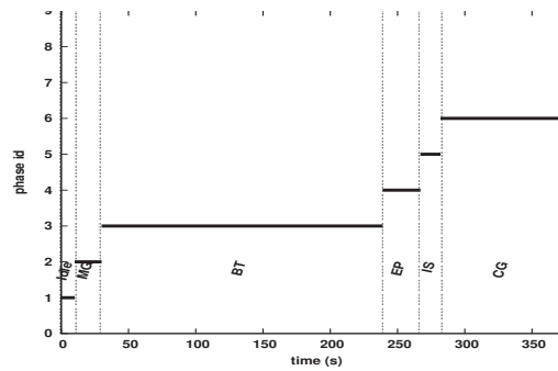
(d) Graphical view of system phase distributions (slave node).
