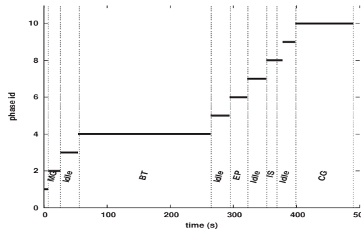
(d) Graphical view of system phase distributions (slave node).
