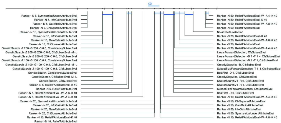
FIG. 1 – Résultats du test de Nemenyi sur les méthodes de sélections d’attributs employées au méta-niveau. Les méthodes sont classées par performance croissante et les groupes connectés ne sont pas jugés significativement différents.
